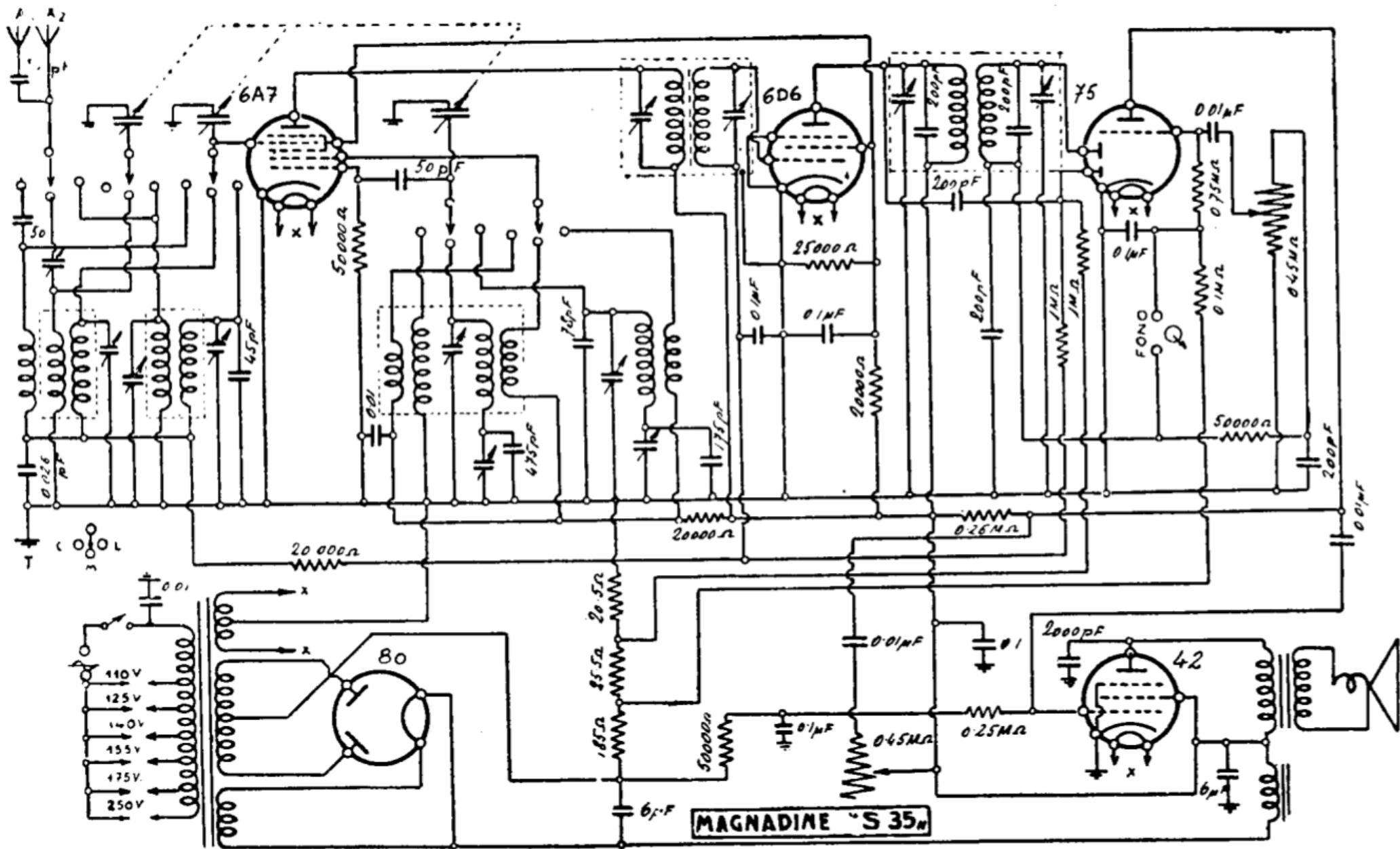
MAGNADYNE RADIO. — Mod. « S 35 ». — Produzione 1936. — Media frequenza: 382.5 kHz.
